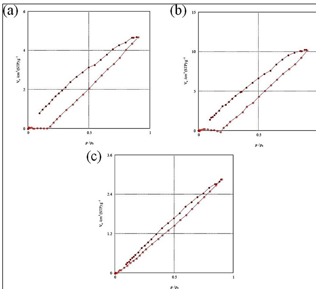
Fig. 5. Nitrogen absorption-desorption isotherm of a) \text{TiO}_2 , b) \text{TiO}_2\text{-CS} , and c) \text{TiO}_2\text{-CS-Ag}
