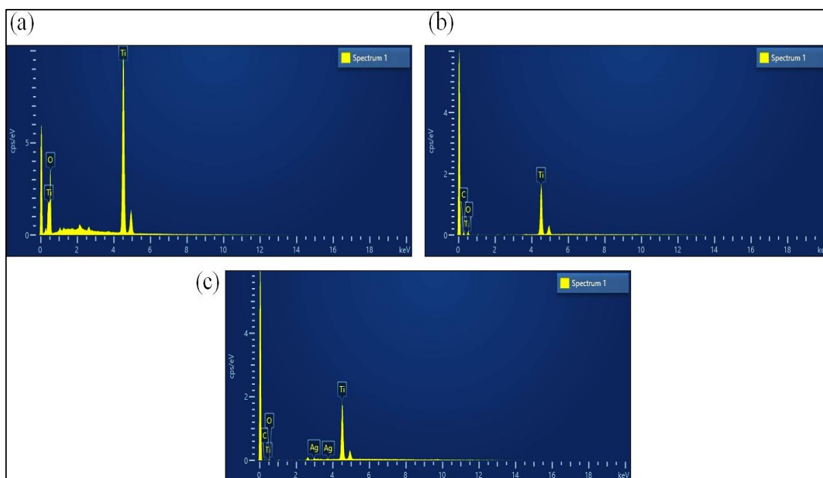
Fig. 4. The EDXS patterns of a) \text{TiO}_2 , b) \text{TiO}_2\text{-CS} , and c) \text{TiO}_2\text{-CS-Ag}
